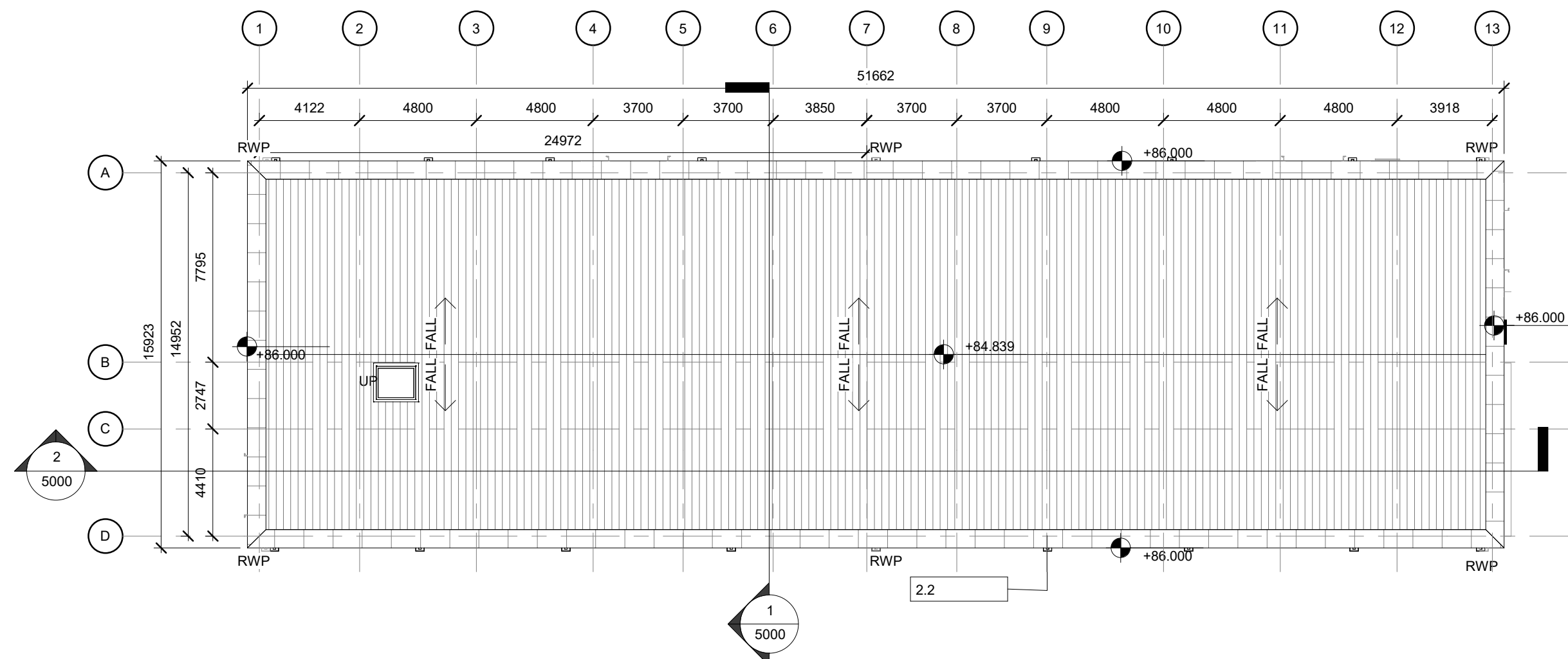
3 ROOF PLAN 1 : 200
